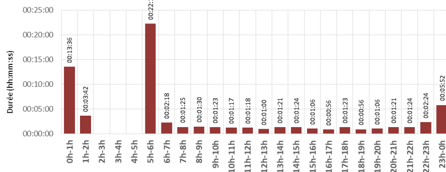
Intervalle entre deux trains - moyenne par heure et en exploitation 75012-PARIS-CORIOLIS
