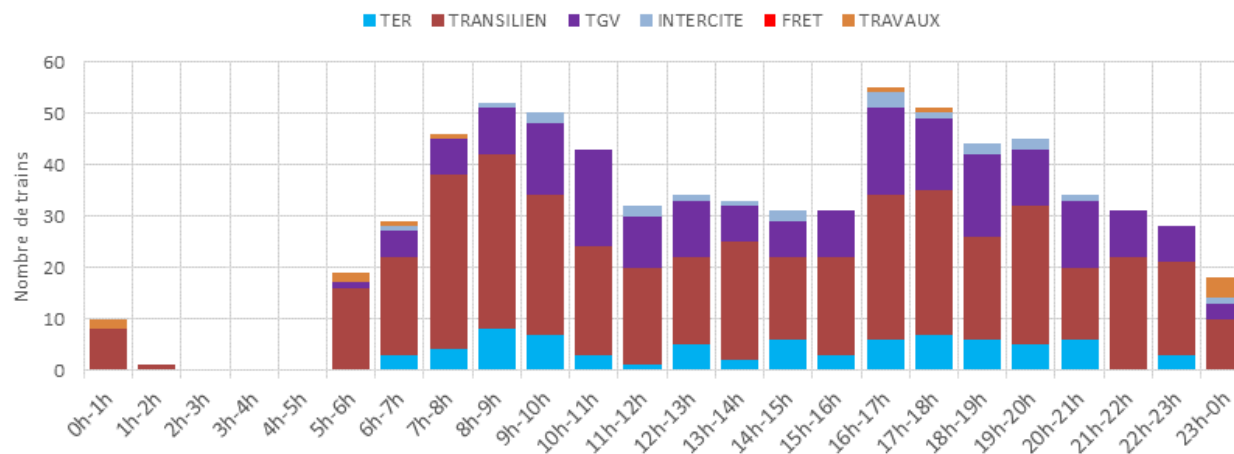
Trafic ferroviaire horaire et répartition par type de circulation 75012-PARIS-CORIOIS
