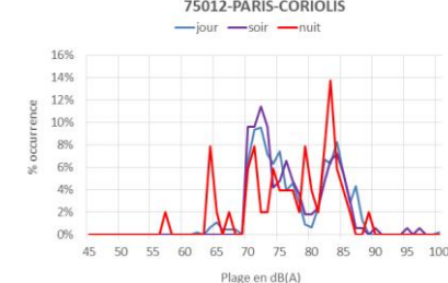
Distribution des L Amax par plages de 1 dB 75012-PARIS-CORIOLIS
