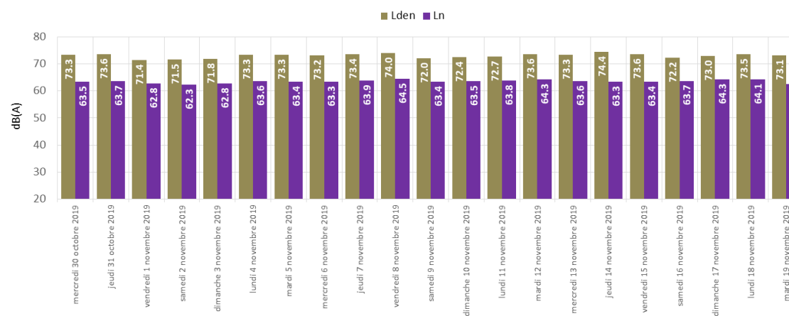
Évolution journalière du bruit ambiant 75012-PARIS-CORLIOLIS
