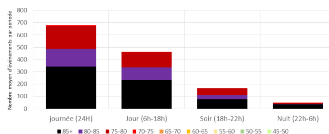
Distribution des SEL - par périodes réglementaires 75012-PARIS-CORIOLIS
