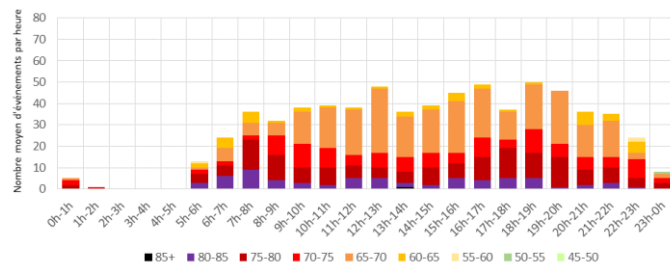
Distribution moyenne horaire des LAeq événements 75012-PARIS-CORIOLIS
