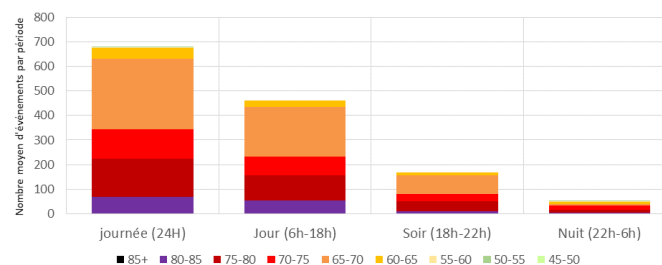
Distribution des LAeq événements - par périodes réglementaires 75012-PARIS-CORIOLIS
