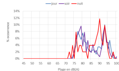
Distribution des SEL par plages de 1 dB 75012-PARIS-CORIOLIS
