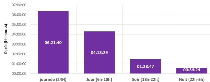
Durée cumulée associée au bruit ferroviaire par périodes 75012-PARIS-CORIOLIS
