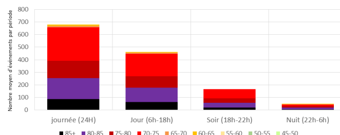
Distribution des L Amax,1s - par périodes réglementaires 75012-PARIS-CORIOLIS
