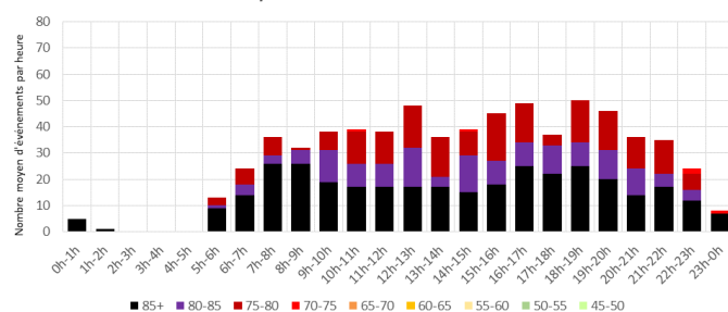
Distribution moyenne horaire des SEL - 75012-PARIS-CORIOLIS
