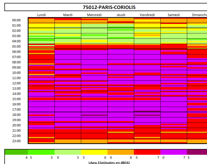
Évolution journalière du bruit ambiant 75012-PARIS-CORLIOLIS
