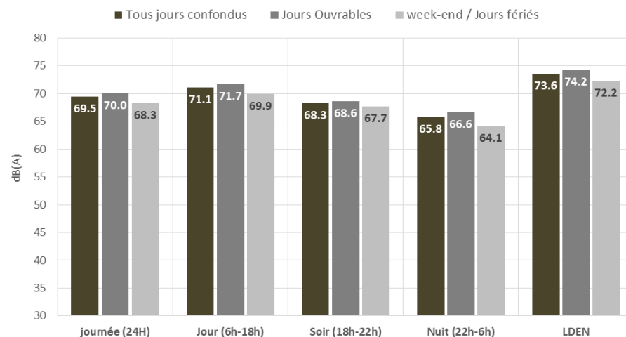
Niveaux de bruit ambiant par périodes et par type de jour 75012-PARIS-CORLIOLIS
