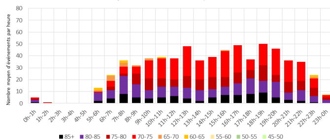
Distribution moyenne horaire des L Amax,1s - 75012-PARIS-CORIOLIS
