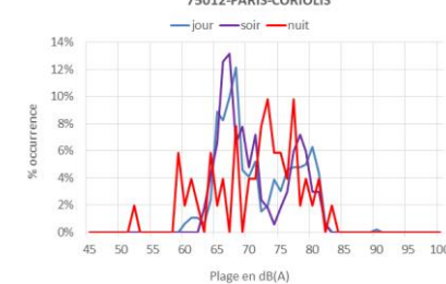
Distribution des LAeq événements par plages de 1 dB 75012-PARIS-CORIOLIS
